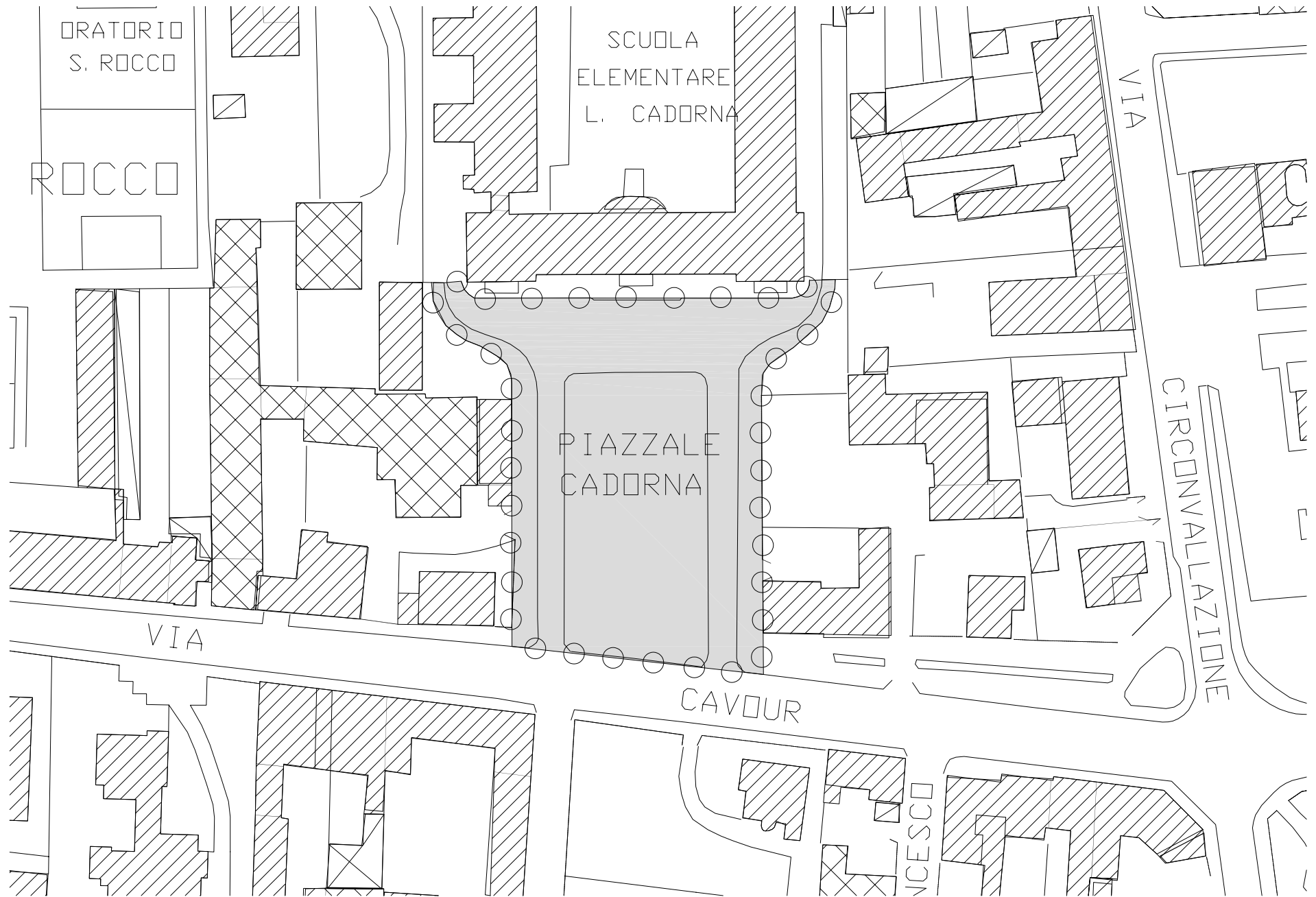
5. Estratto Aereofotogrammetrico, scala 1:1000
